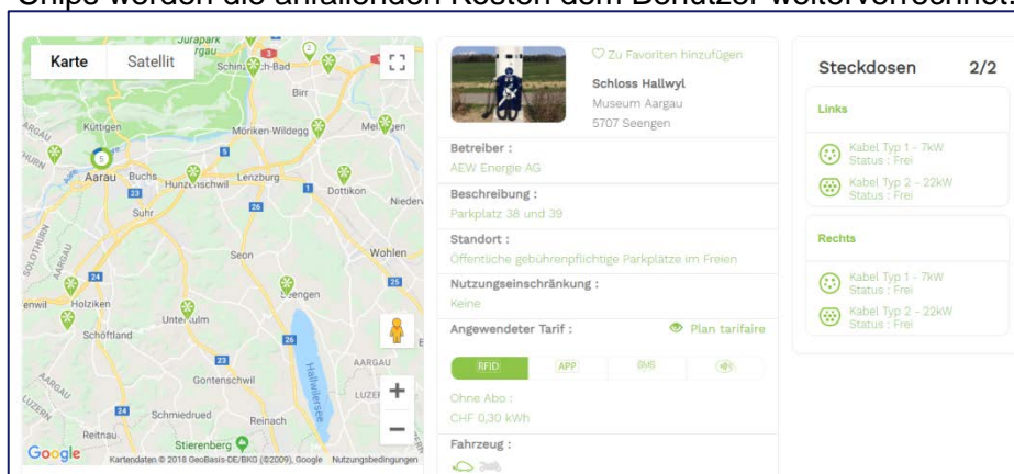
Abbildung 6: EVPass Portal
