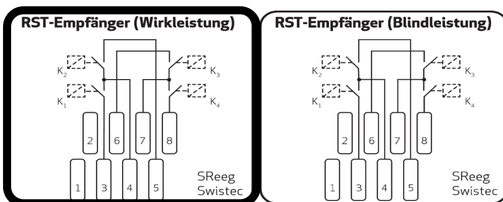
Abbildung 3: Schnittstelle bei der Klemmleiste (RST-Empfänger), Wirkleistung vorgeschrieben, Blindleistung nur vorbereitet
