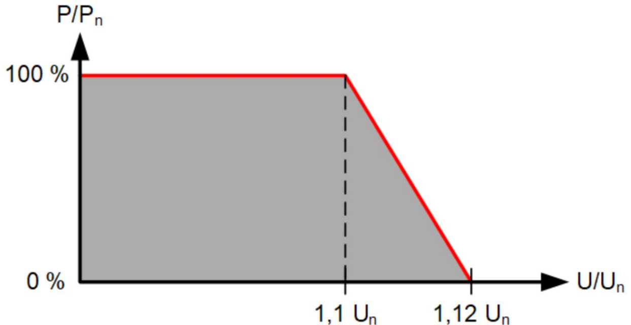
Abbildung 1: P(U)-Kennlinie zur Regelung der Wirkleistung in Abhängigkeit der gemessenen Spannung beim Wechselrichter
