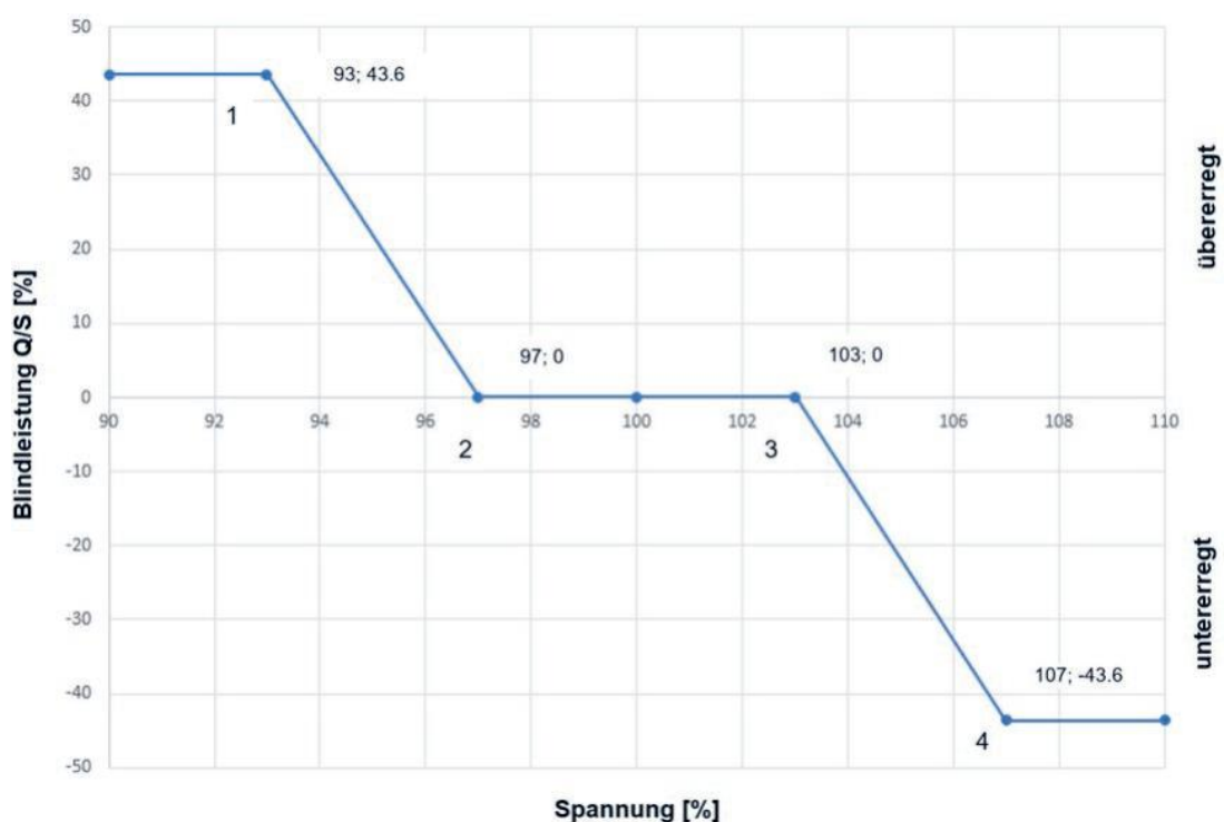
Abbildung 2: Q(U)-Kennlinie im Erzeugerpeilsystem
