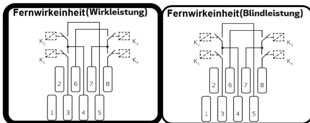
Abbildung 3: Schnittstelle bei der Klemmleiste (Fernwirkeinheit), Wirkleistung vorgeschrieben, Blindleistung nur vorbereitet
