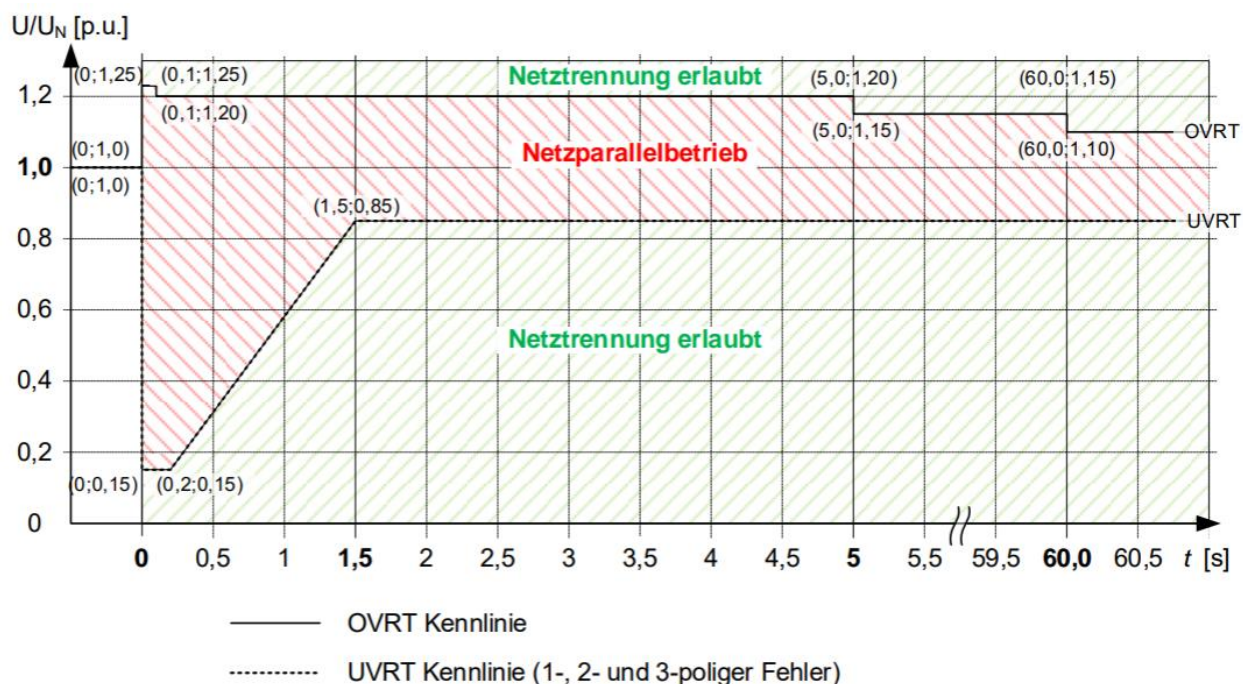
Abbildung 5: u(t)-Kennlinie für FRT-Verhalten von EEA Typ 2 (nichtsynchron) und elektrische Energiespeicher
